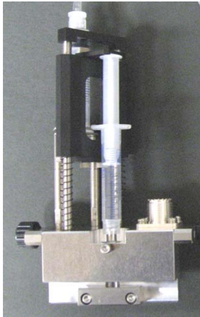
Tube-less Spinneret
